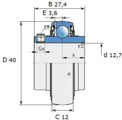
Размеры (мм): LE 201-008 2F
