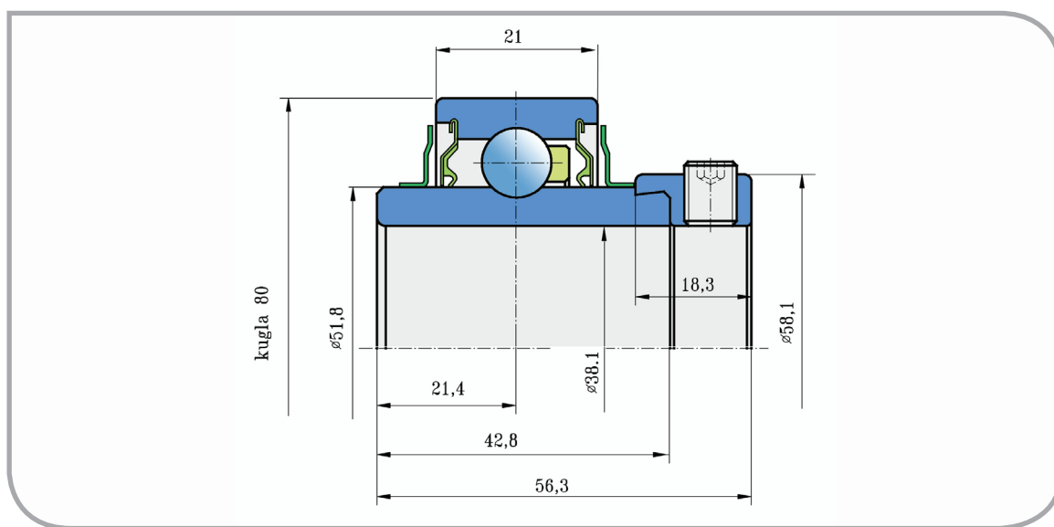
Размеры/Dimensions (mm)
