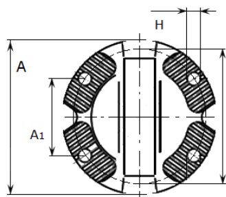
Тип 1. С ТОРЦЕВЫМИ ШЛИЦАМИ
