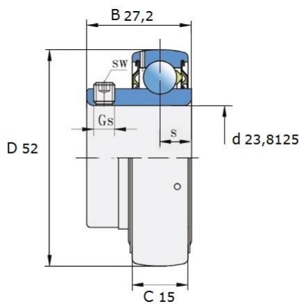
Размеры (мм): UE 205-015 2S
