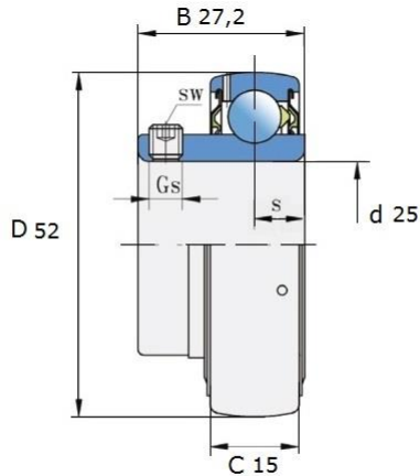
Размеры (мм): UE 205-2S
