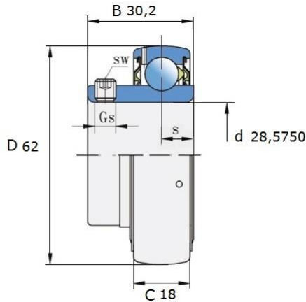
Размеры (мм): UE 206-102 2S
