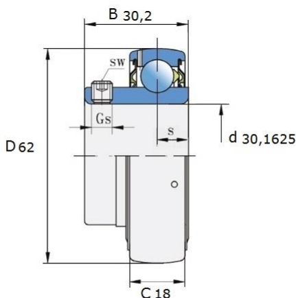
Размеры (мм): UE 206-103 2S
