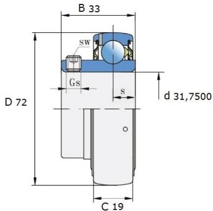
Размеры (мм): UE 207-104 2S
