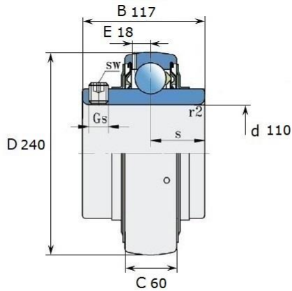
Размеры (мм): LE 322 2F
