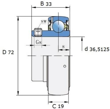
Размеры (мм): UE 207-107 2S
