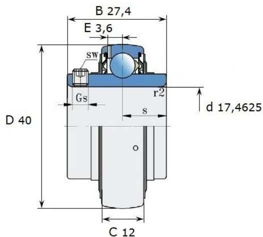
Размеры (мм): LE 203-011 2F
