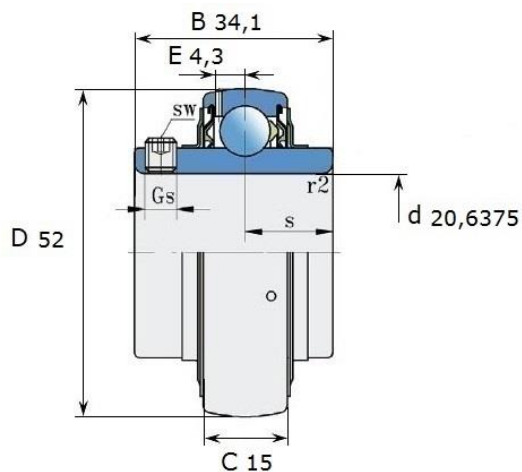
Размеры (мм): LE 205-013 2F
