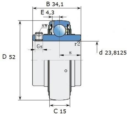
Размеры (мм): LE 205-015 2F
