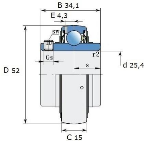
Размеры (мм): LE 205-100 2F
