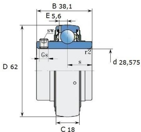
Размеры (мм): LE 206-102 2F
