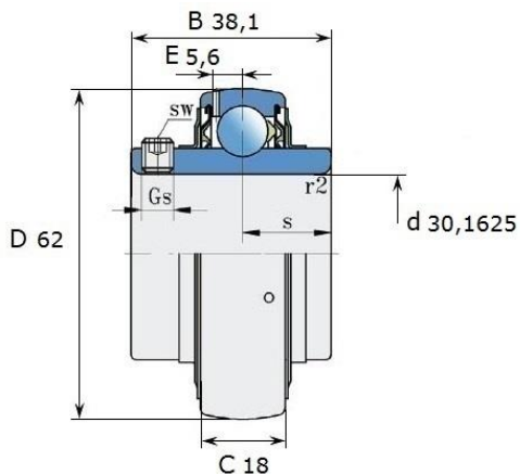
Размеры (мм): LE 206-103 2F
