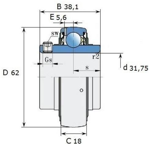
Размеры (мм): LE 206-104 2F
