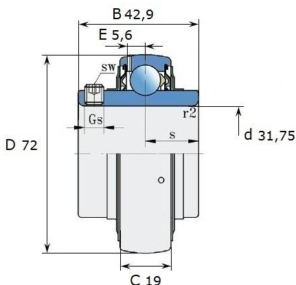
Размеры (мм): LE 207-104 2F
