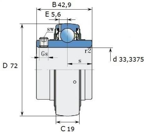
Размеры (мм): LE 207-105 2F
