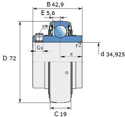
Размеры (мм): LE 207-106 2F
