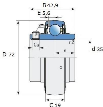
Размеры (мм): LE 207 2F
