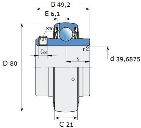
Размеры (мм): LE 208-109 2F
