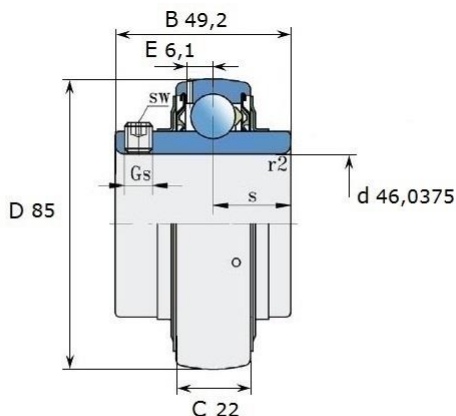
Размеры (мм): LE 209-113 2F
