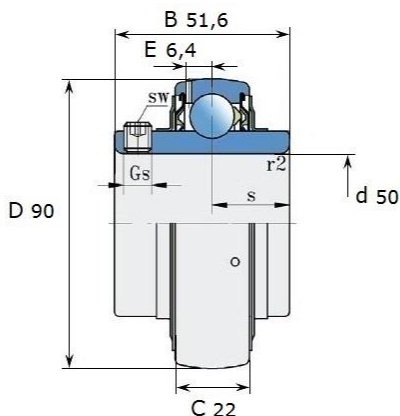
Размеры (мм): LE 210 2F
