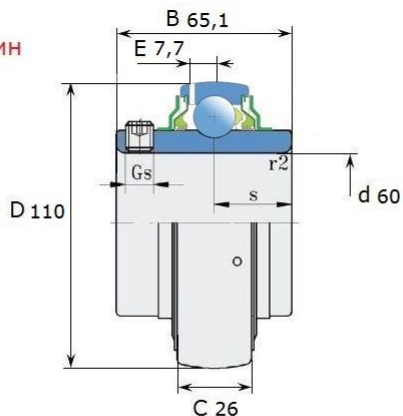
Размеры (мм): LE 212 2ТВ
