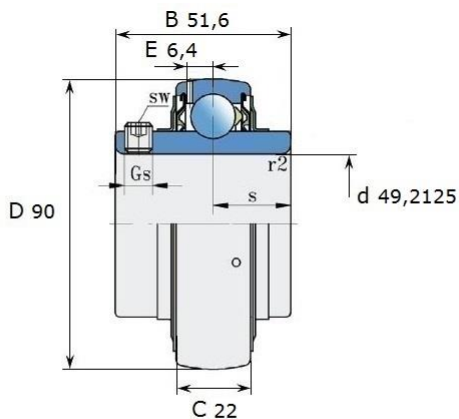
Размеры (мм): LE 210-115 2F
