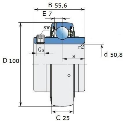
Размеры (мм): LE 211-200 2F
