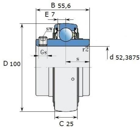
Размеры (мм): LE 211-201 2F
