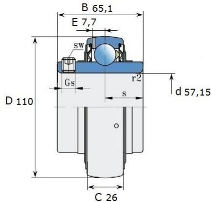
Размеры (мм): LE 212-204 2F
