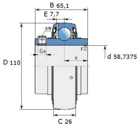
Размеры (мм): LE 212-205 2F
