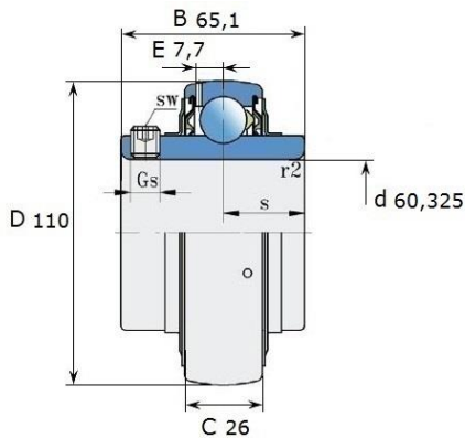
Размеры (мм): LE 212-206 2F
