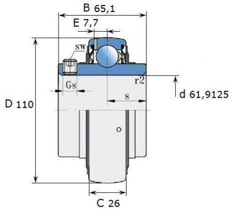
Размеры (мм): LE 212-207 2F
