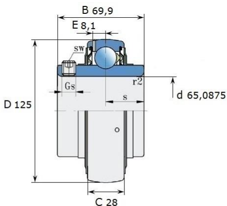
Размеры (мм): LE 214-209 2F
