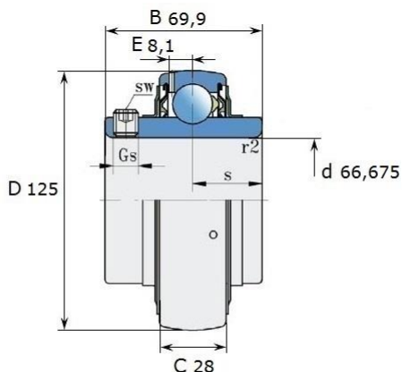
Размеры (мм): LE 214-210 2F
