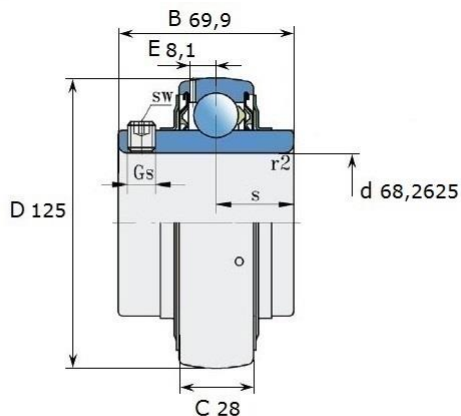
Размеры (мм): LE 214-211 2F
