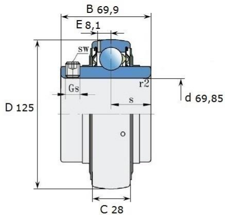
Размеры (мм): LE 214-212 2F
