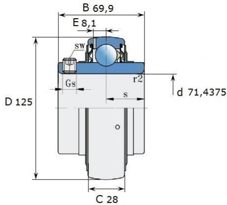
Размеры (мм): LE 214-213 2F
