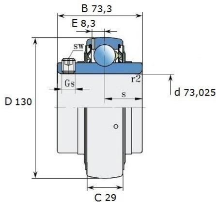
Размеры (мм): LE 215-214 2F
