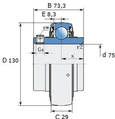
Размеры (мм): LE 215 2F
