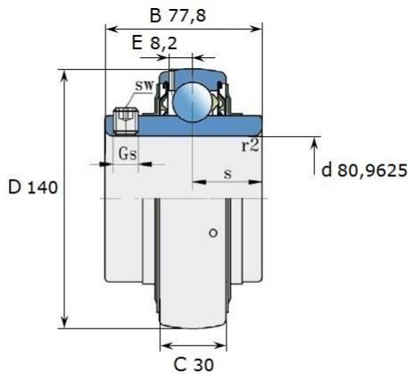
Размеры (мм): LE 216-303 2F
