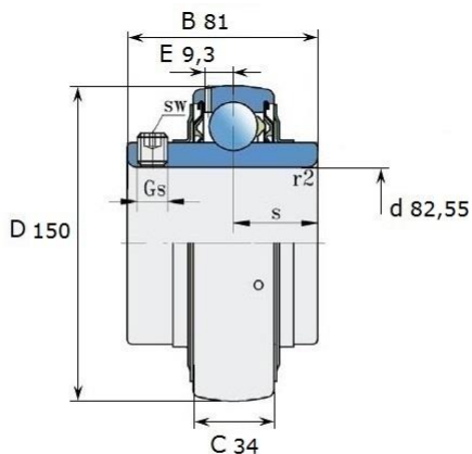
Размеры (мм): LE 217-304 2F
