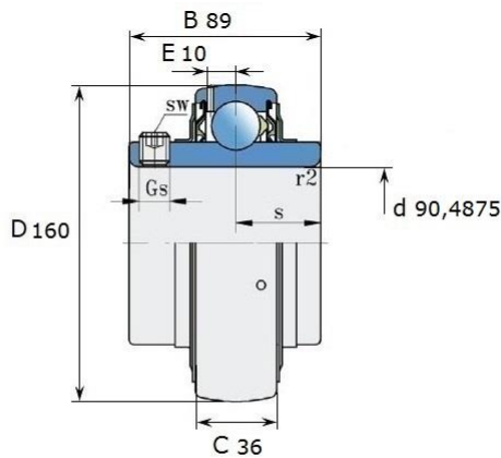
Размеры (мм): LE 218-309 2F
