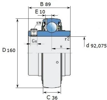
Размеры (мм): LE 218-310 2F
