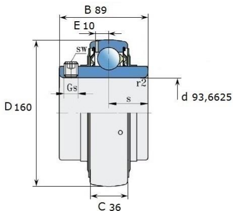
Размеры (мм): LE 218-311 2F
