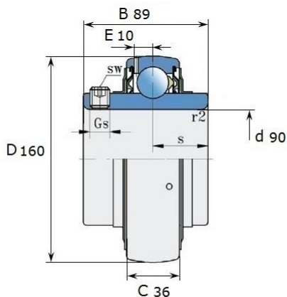
Размеры (мм): LE 218 2F
