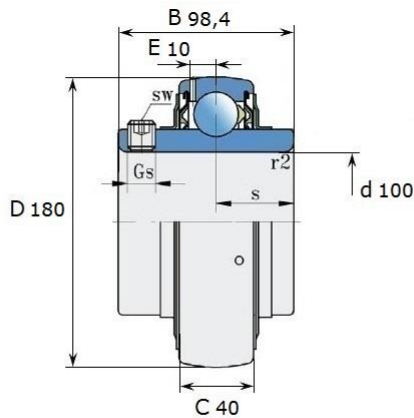
Размеры (мм): LE 220 2F
