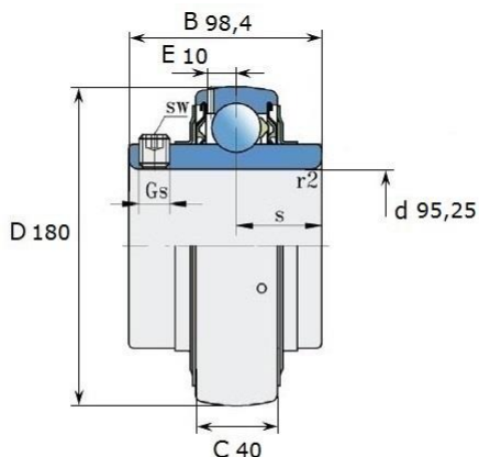
Размеры (мм): LE 220-312 2F
