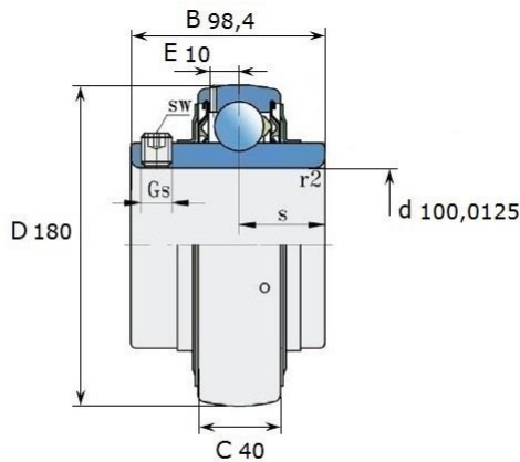
Размеры (мм): LE 220-315 2F
