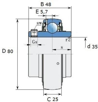
Размеры (мм): LE 307 2F
