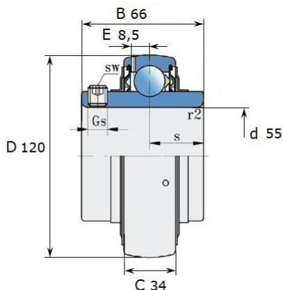
Размеры (мм): LE 311 2F
